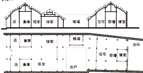
ホイアンの町家の空間構成 (昭和女子大学国際文化研究所紀要 Vol.3 『ベトナム・ホイアンのまち並みと建築』(1996)より)
