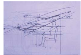
新幹線先端形状を決める為の運転席断面検討 (提供：(株)剣持デザイン研究所)
